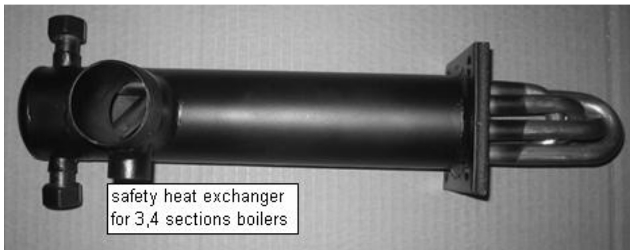
Б Теплообменник безопасности для 3-х и 4-х секционного котла
