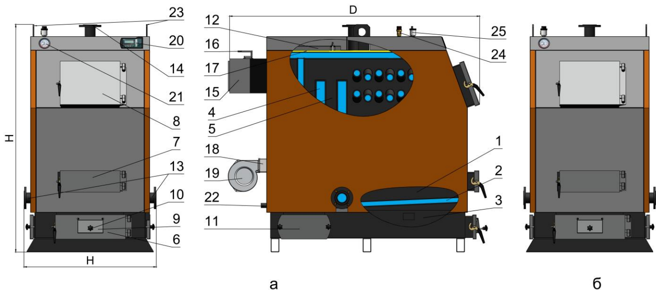
Рисунок 1 - Будова котла типу KV*, де:
