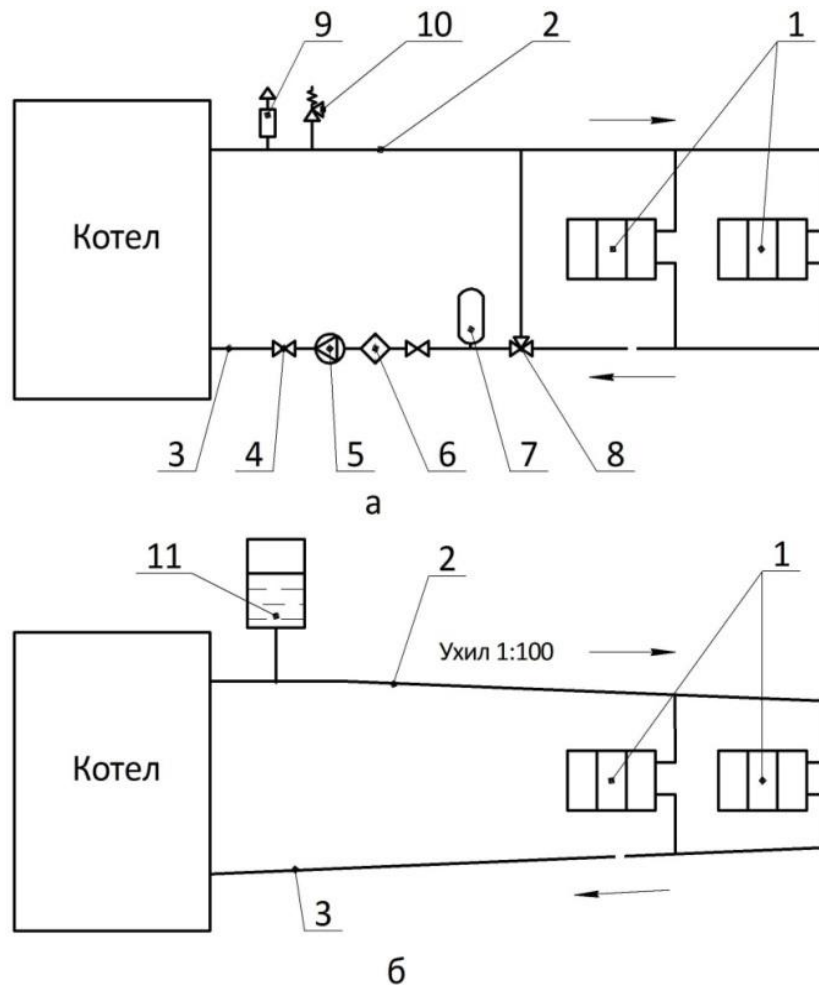
Рисунок 4 - Схеми підключення котла до системи опалення:
