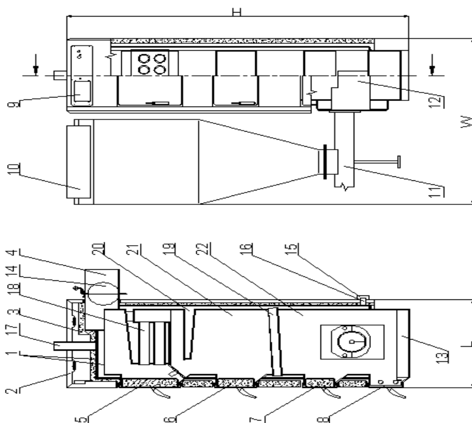
Rys. Kocioł SD
